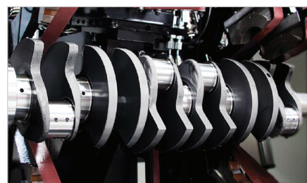
Superfinišování klikové hřídele na stroji CenFlex 1
