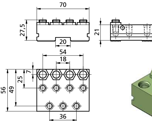
PCZB7021PRF kg ~0,6
