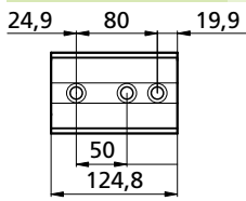
PCB50320H80 kg ~14,3
