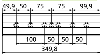
PCB50400H80 kg ~18,1
