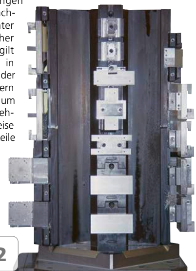
Kleinserienfertigung auf Horizontalmaschinen: Autarke Spannstellen ermöglichen die gleichzeitige, spezifische Fixierung unterschiedlicher Werkstücke.
