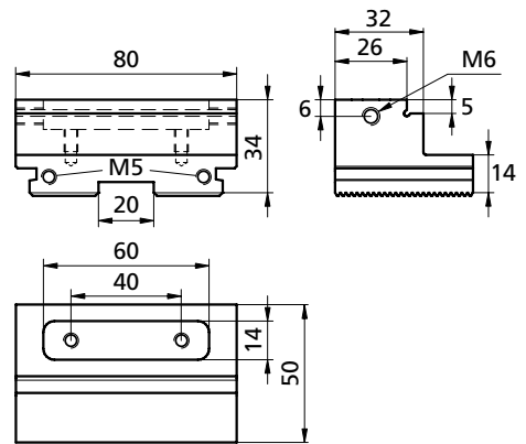
PCZB7023PRG kg ~0,54
