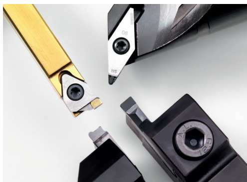
Diamantové soustružnické nástroje Horn
